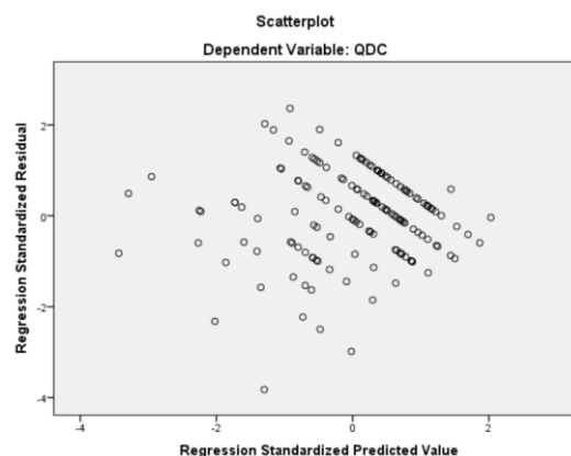
Hình 3.3: Biểu đồ Scatter Plot
