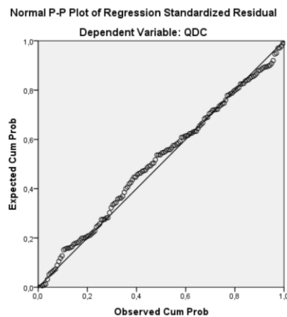
Hình 3.2: Biểu đồ P-P Plot
