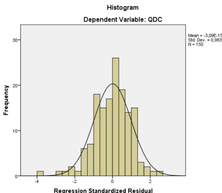
Hình 3.1: Sơ đồ Histogram
