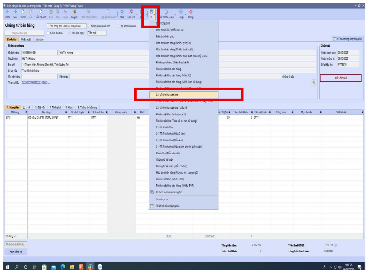
Hình 2.24 : Giao diện chứng từ bán hàng để lấy phiếu xuất kho trên phần mềm MISA
