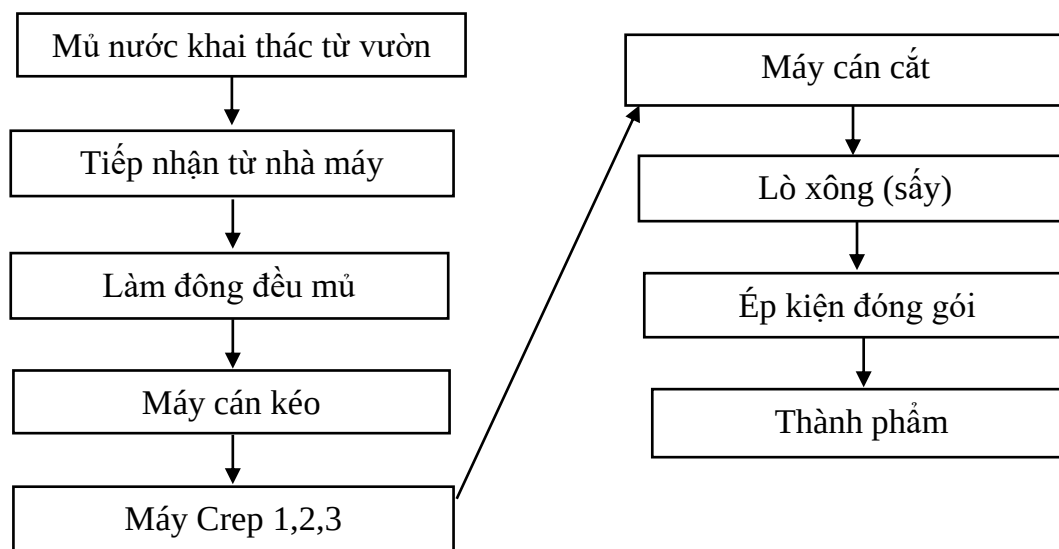
Sơ đồ 2.1 Quy trình công nghệ sản xuất mủ cao su
