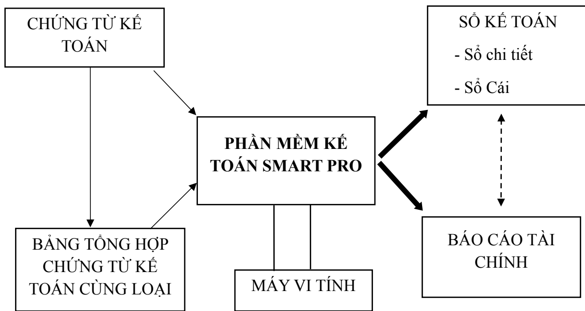
Sơ đồ 2.4. Sơ đồ trình tự ghi sổ kế toán theo trên phần mềm Smart Pro
